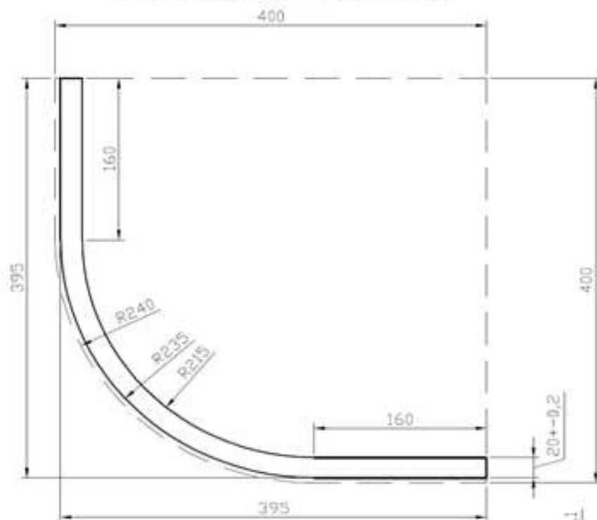
F01-F02 HAJLÍTOTT (400x400)
