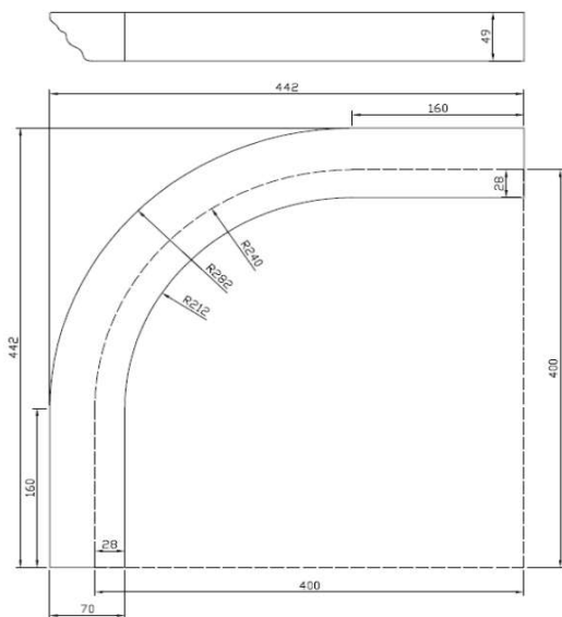
PAR01 HAJLÍTOTT (400x400)
