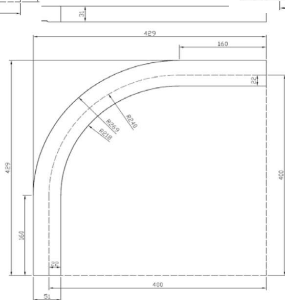
PAR02 HAJLÍTOTT (400x400)
